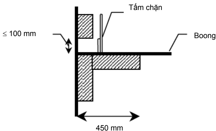
Hình 5/2.3 Lớp bọc chống cháy cho chân vách
